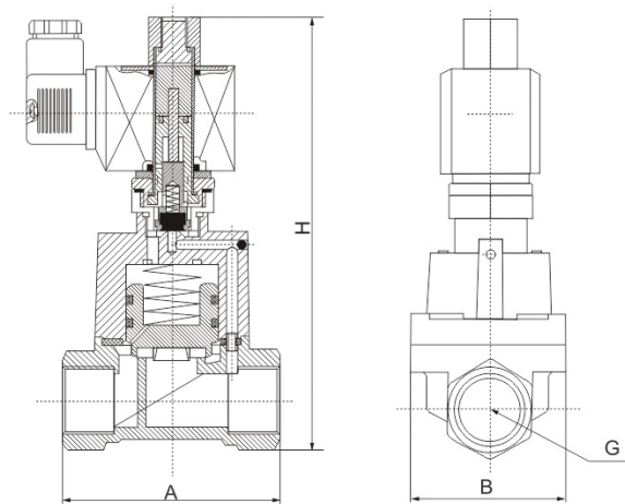
外形简图
