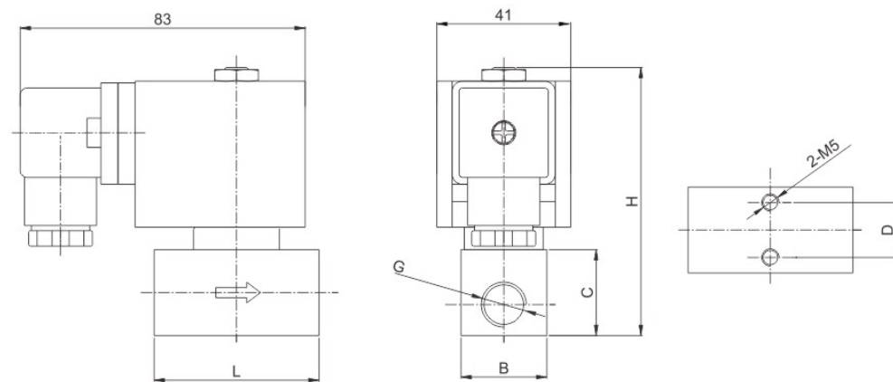
外形简图
