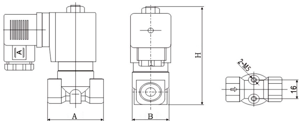
外形简图
