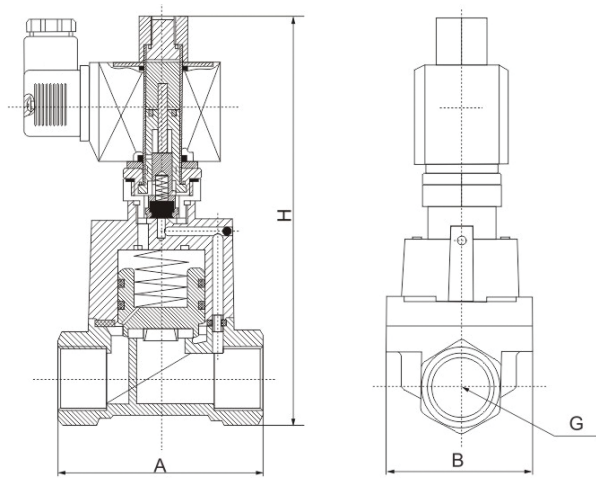
外形简图
