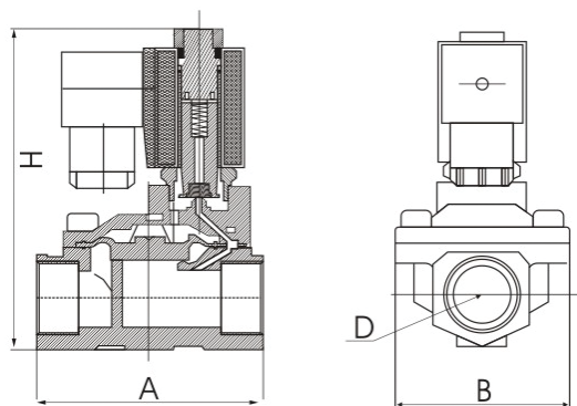
外形简图
