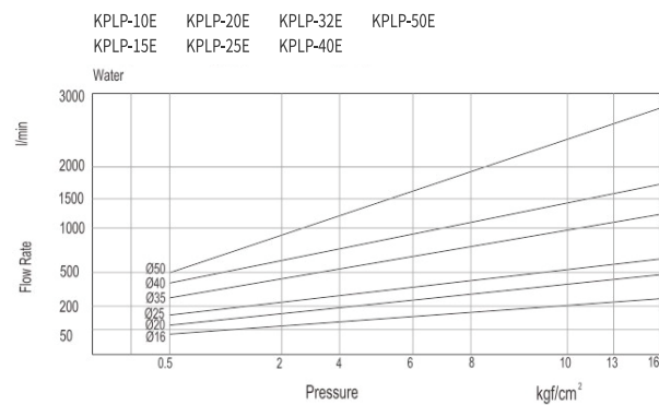
流量线图
