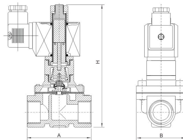
外形简图
