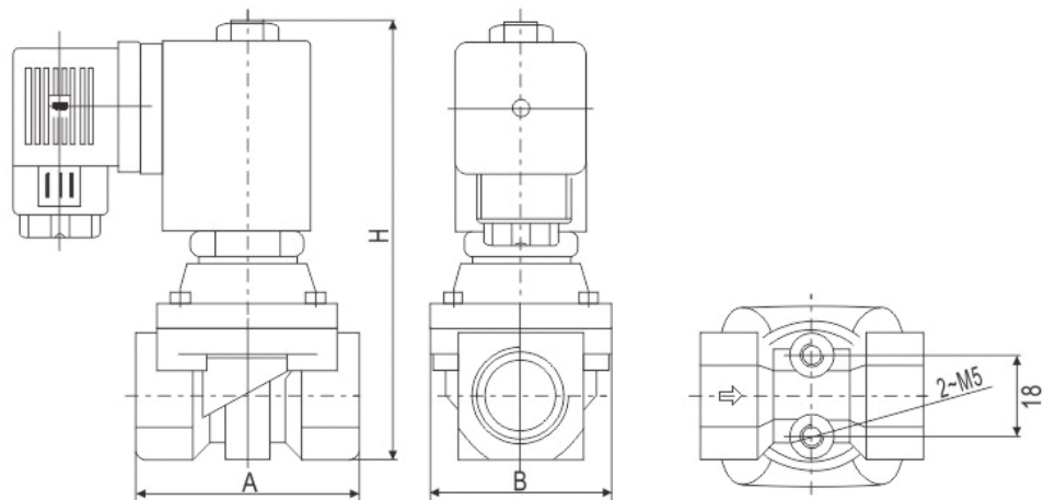
外形简图
