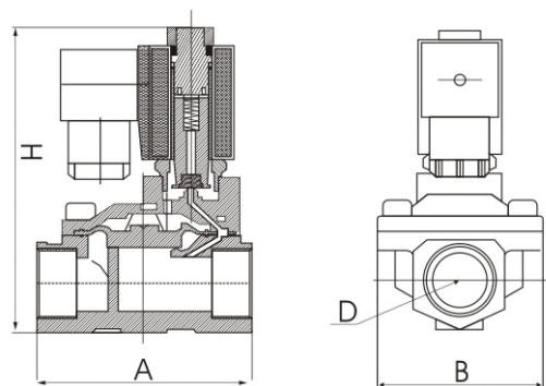
外形简图
