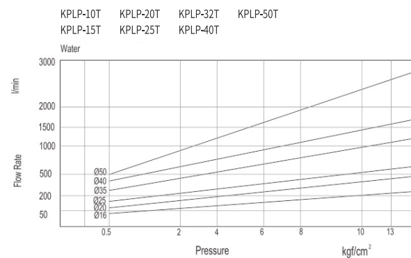
流量线图
