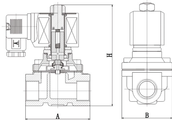
外形简图
