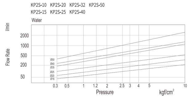
流量线图
