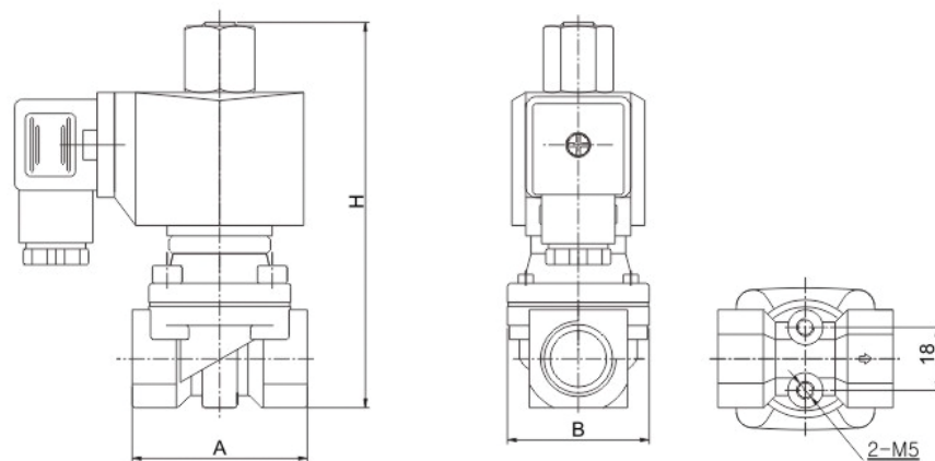
外形简图
