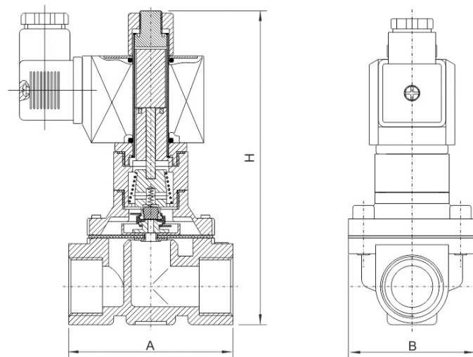
外形简图
