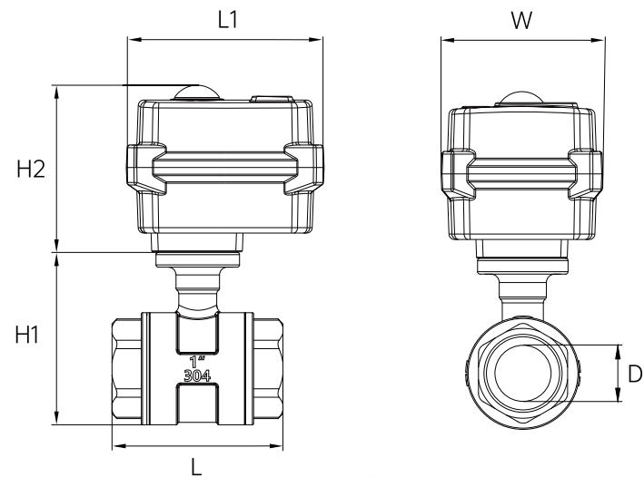
外形简图
