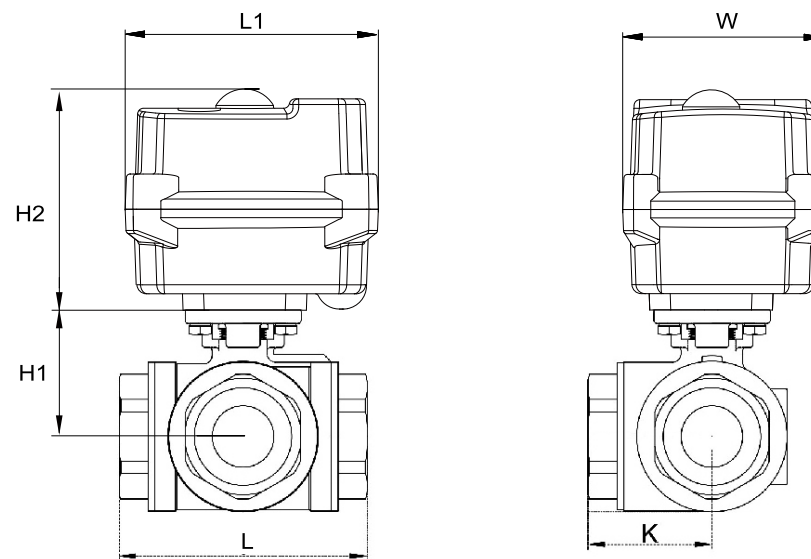
外形简图
