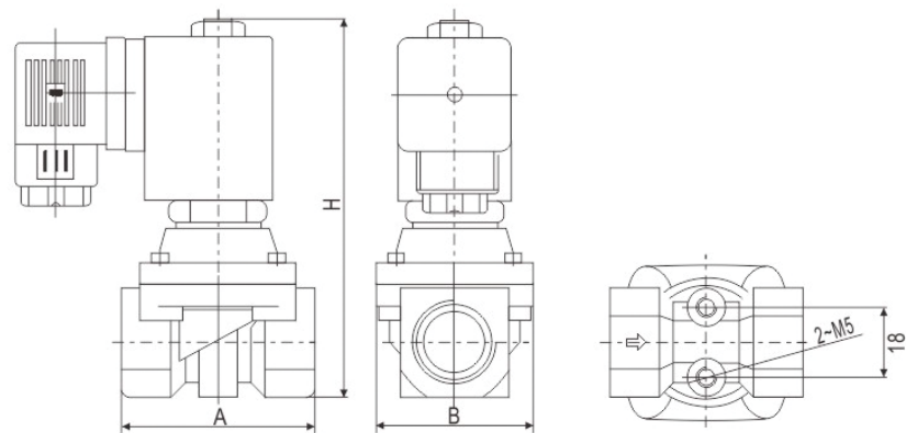
外形简图
