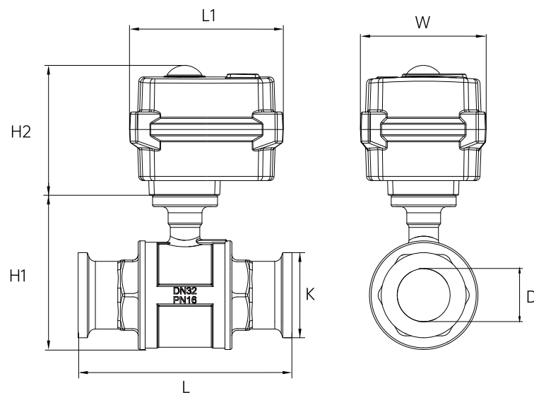
外形简图
