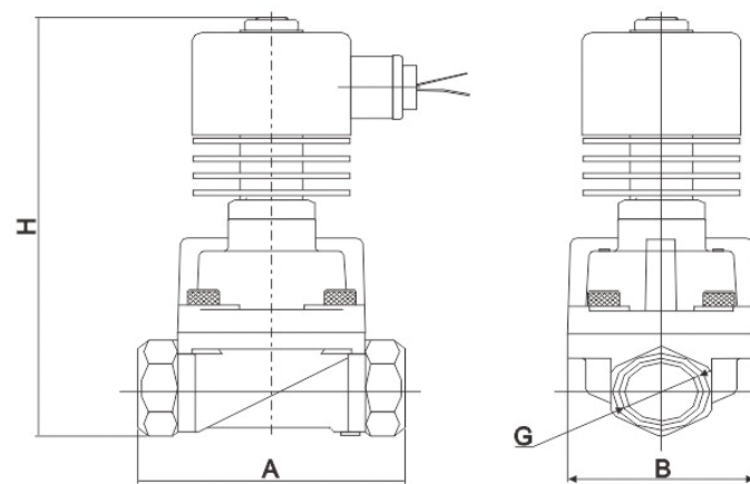
外形简图
