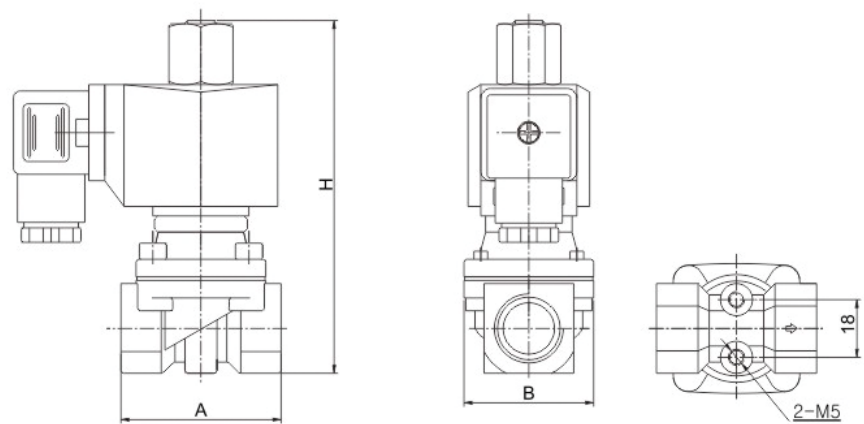
外形简图
