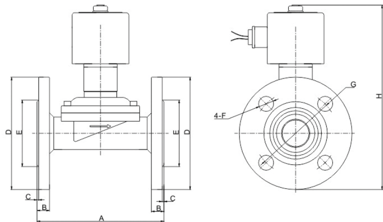
外形简图
