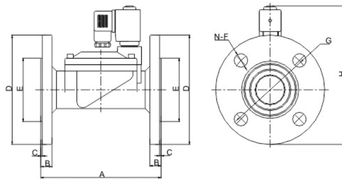
外形简图
