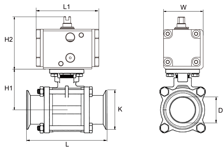
外形简图
