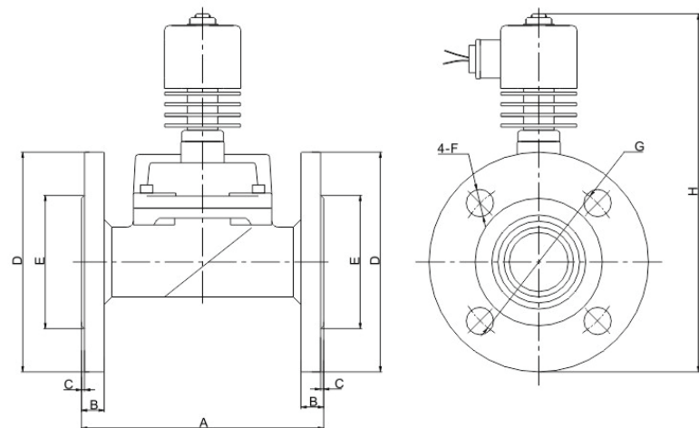
外形简图
