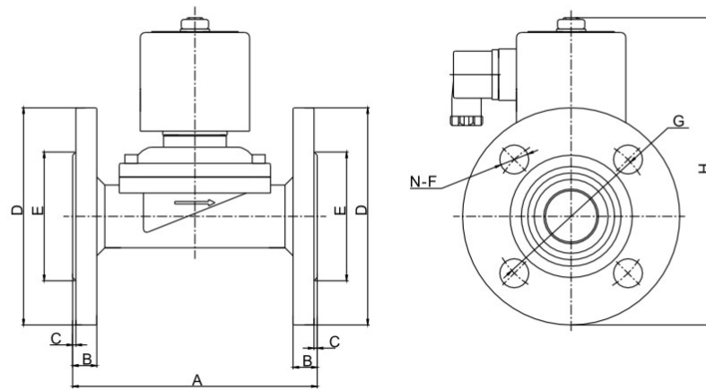
外形简图
