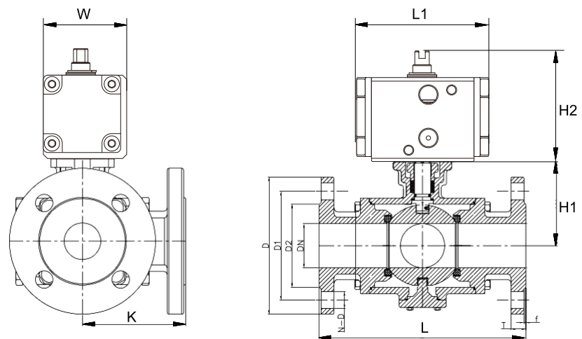
外形简图
