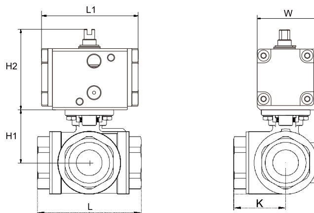
外形简图
