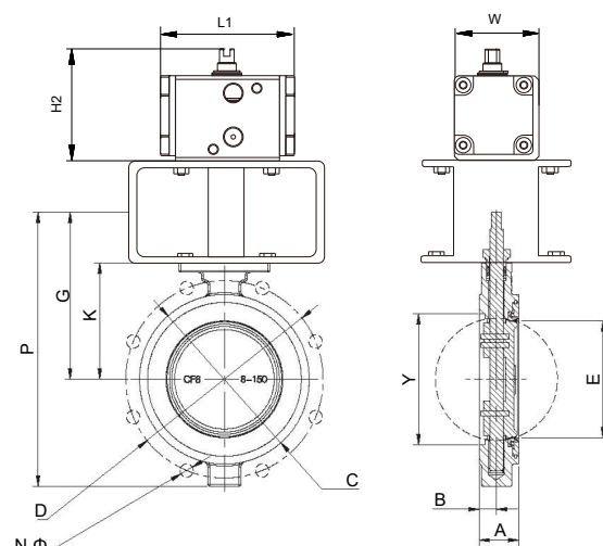
外形简图
