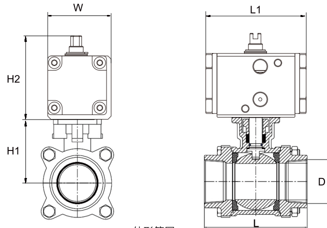
外形简图
