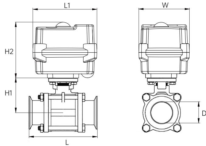
外形简图
