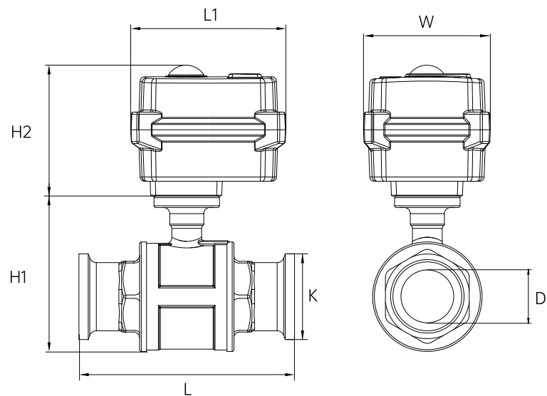
外形简图
