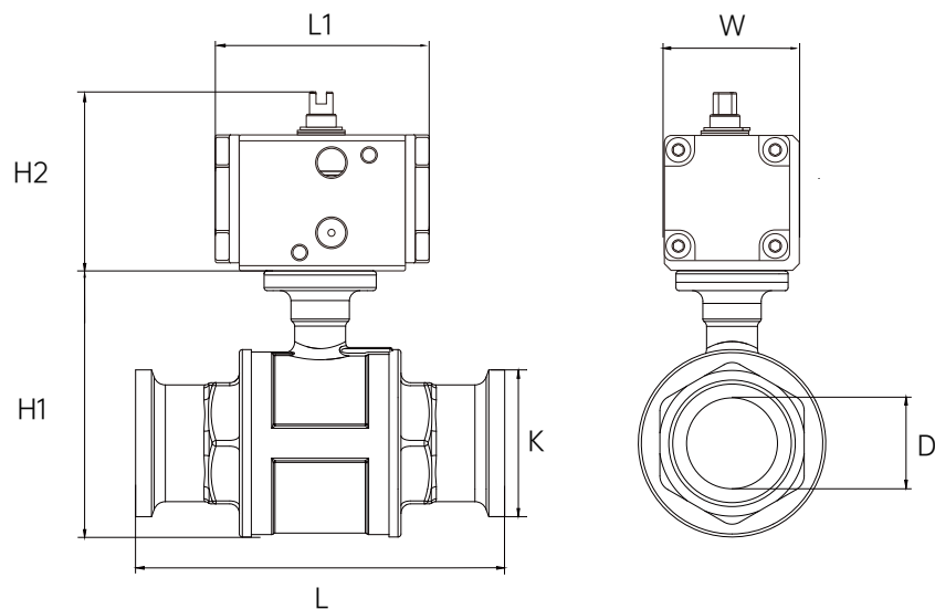
外形简图
