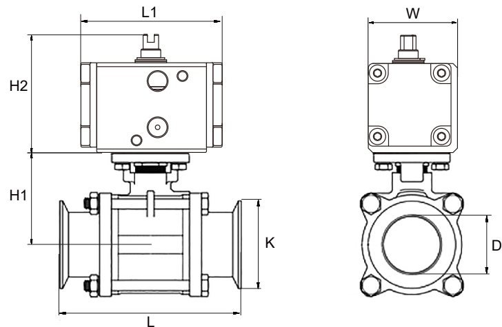
外形简图
