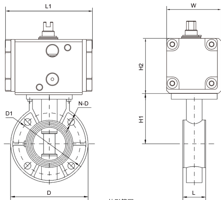
外形简图
