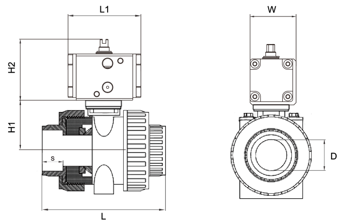
外形简图
