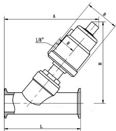
外形简图
