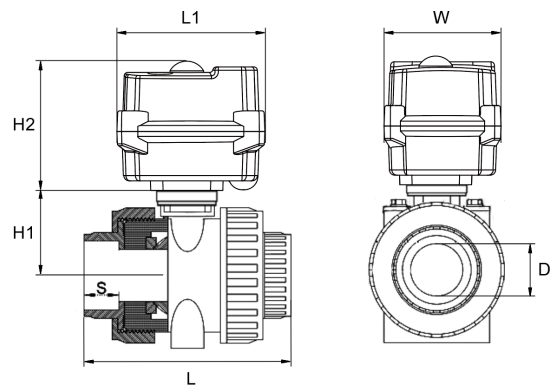
外形简图
