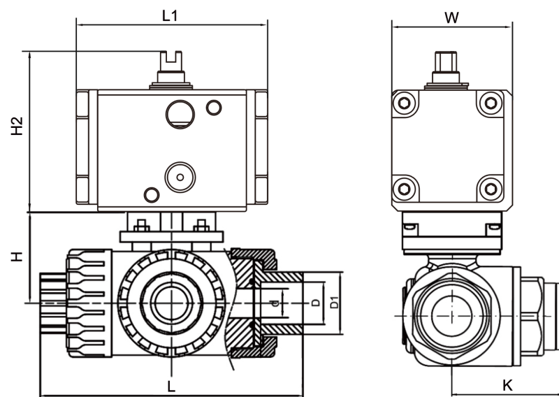
外形简图
