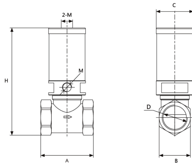
外形简图
