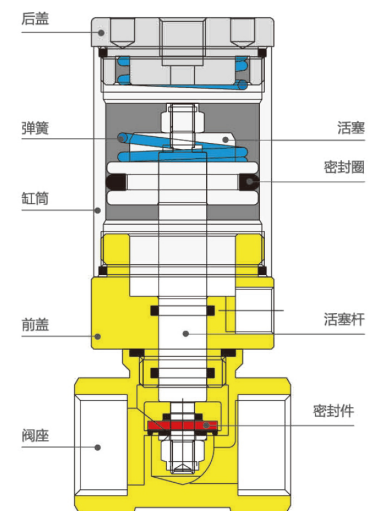
外形剖面图
