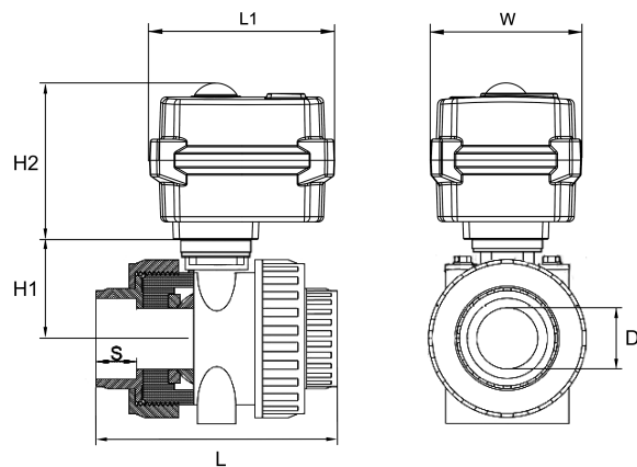
外形简图
