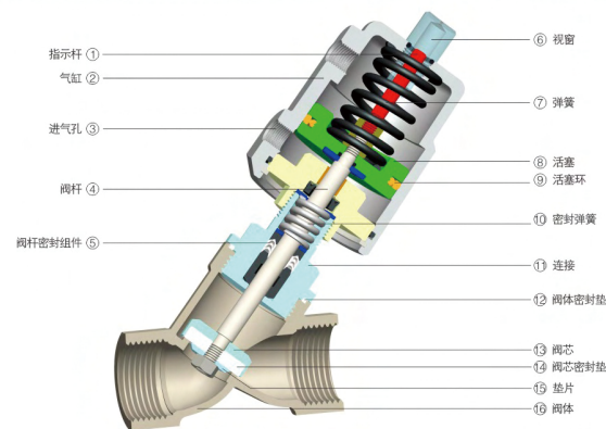
外形剖面图
