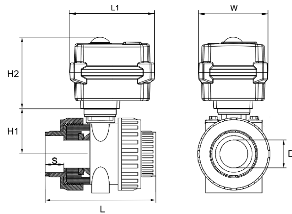
外形简图
