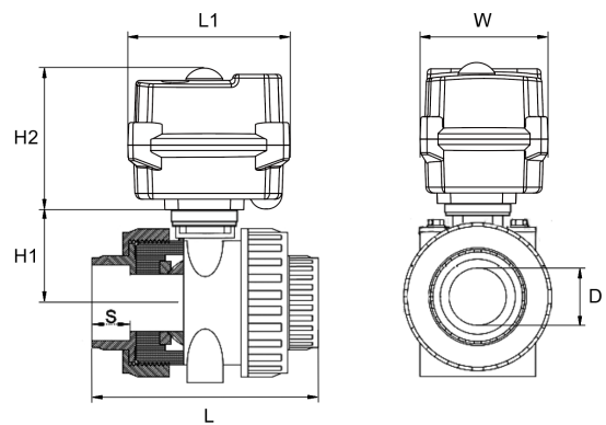
外形简图
