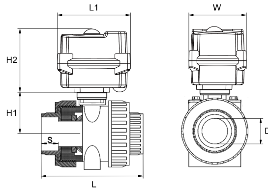
外形简图
