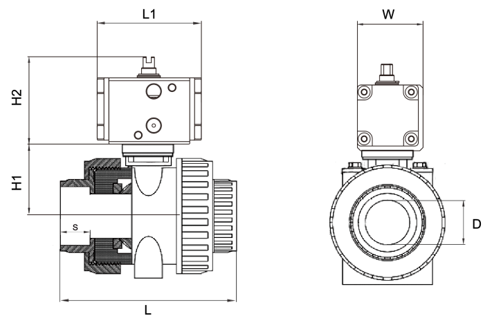
外形简图
