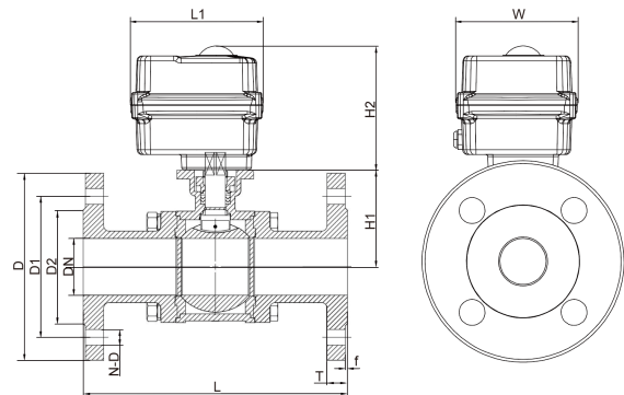
外形简图
